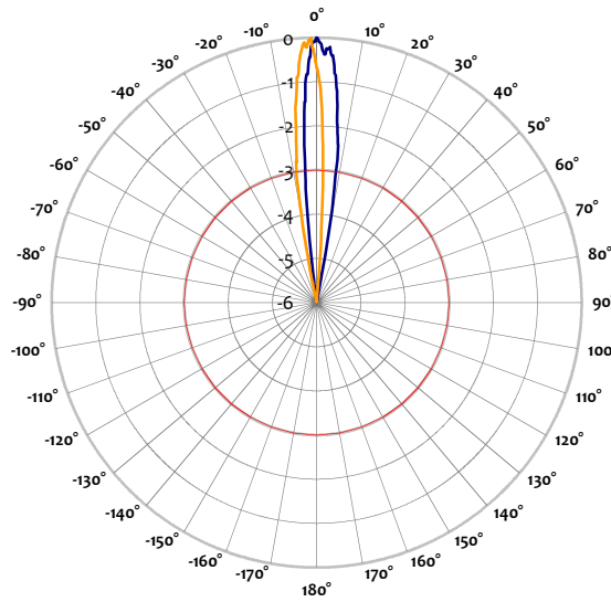
3 dB Beamwidth
