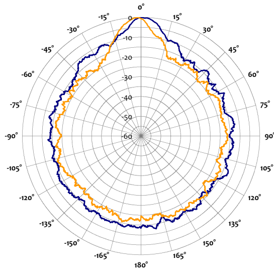
3 dB Beamwidth
